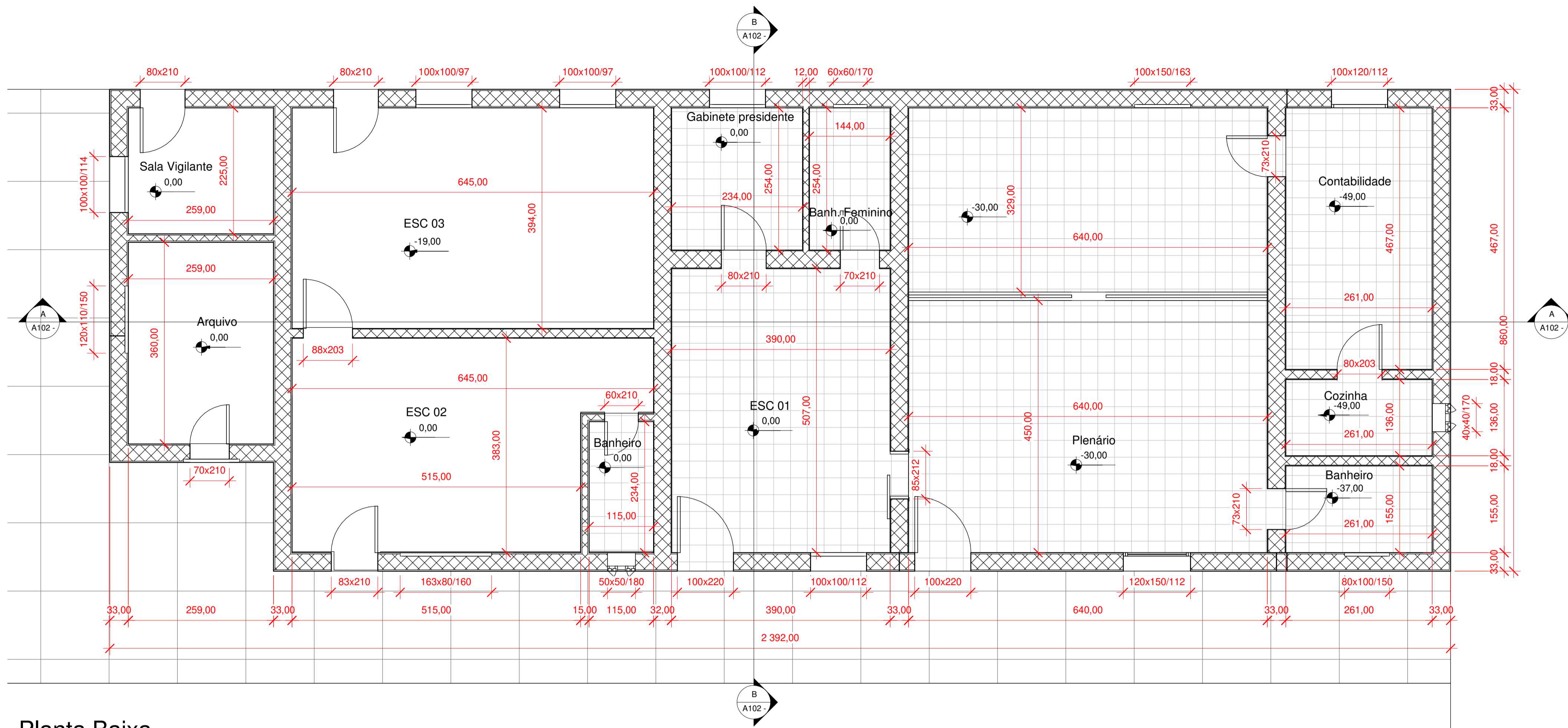
A Planta Baixa 1 : 50
