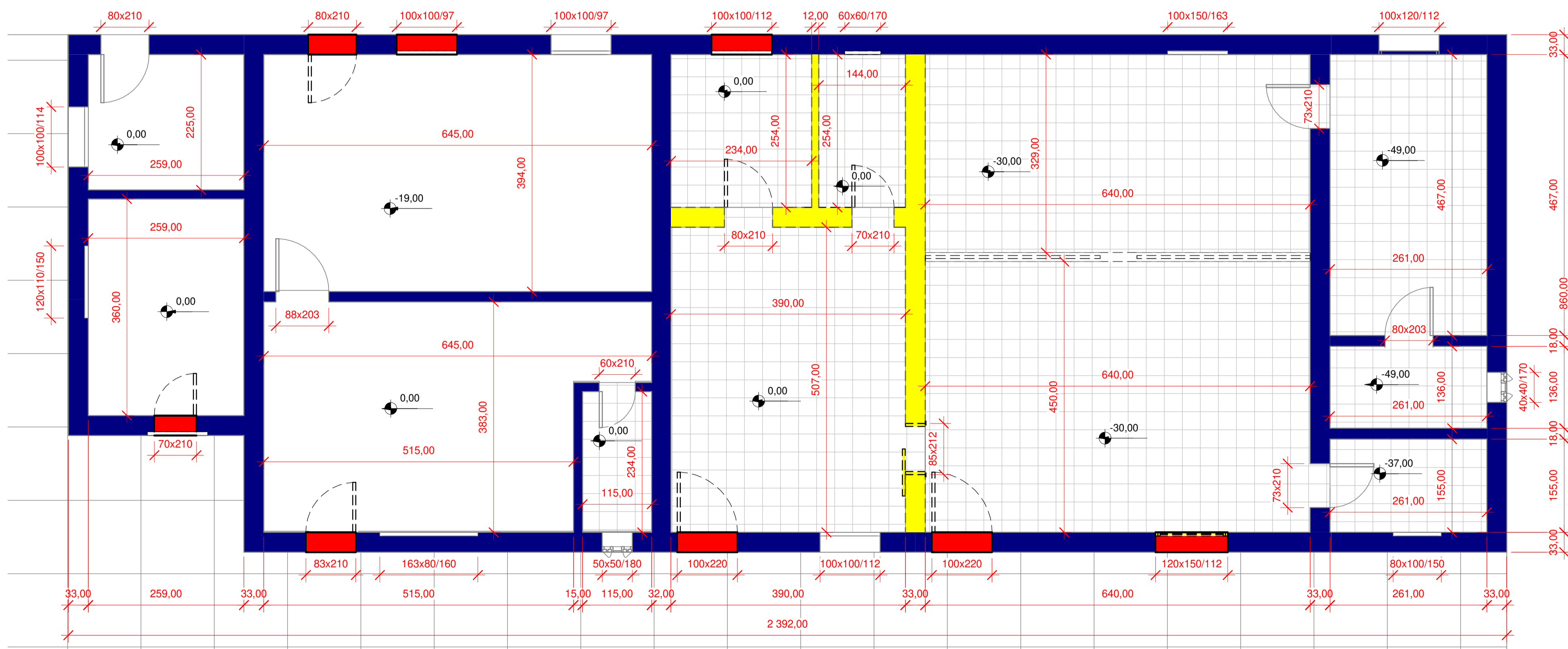
2 Planta de Demolição 1 : 50
